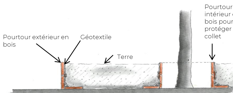
Coupe de principe d'un entourage
